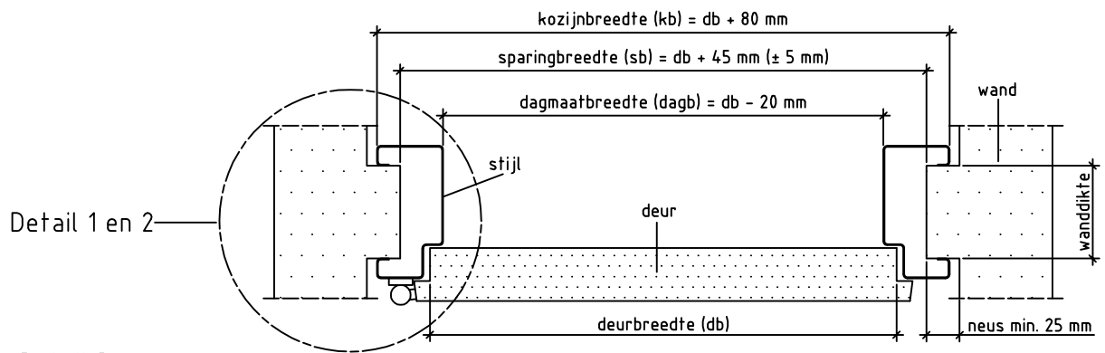
Doorsnede AA
